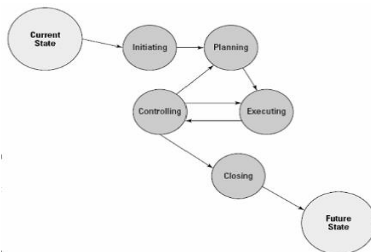
Gambar 1. Tahapan-tahapan Proyek [7]
